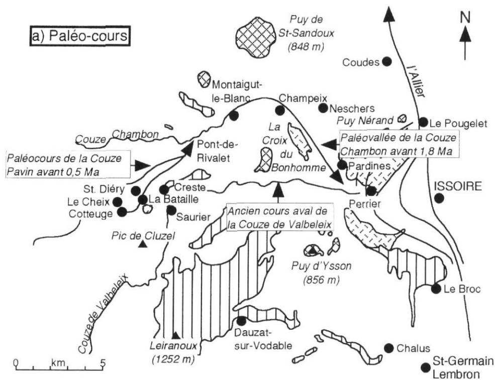
FIGURE 8. Modifications de tracés hydrographiques dans la région des Couzes Modifications of the courses of the Couzes rivers.
