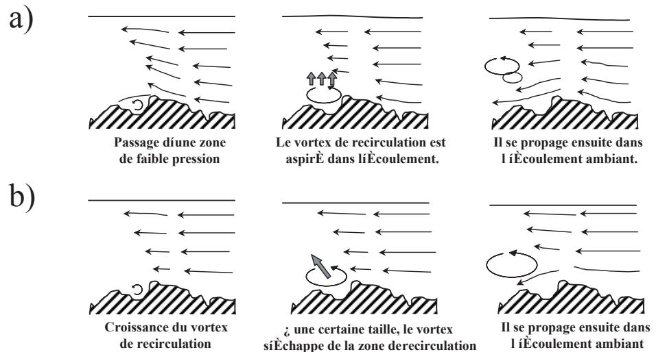
FIGURE 5. Illustration de mécanismes d'échappement à partir (a) des changements de pression de l'écoulement ambiant et (b) de la dynamique interne de la zone de recirculation (d'après Kirkbride, 1993). Ces deux mécanismes sont liés aux passages des structures à grande échelle.
