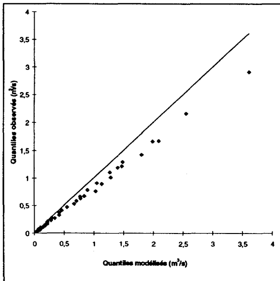
Figure 22 Crisu-Alb à CRISCIOR « QCN(T, d) ». Crisu-Alb's basin at CRISCIOR "QCN(T, d)". ( D_e = 10,4 j et VCN(2, 1) = 0,204 m 3 /s) – Nash% : 90,9.
