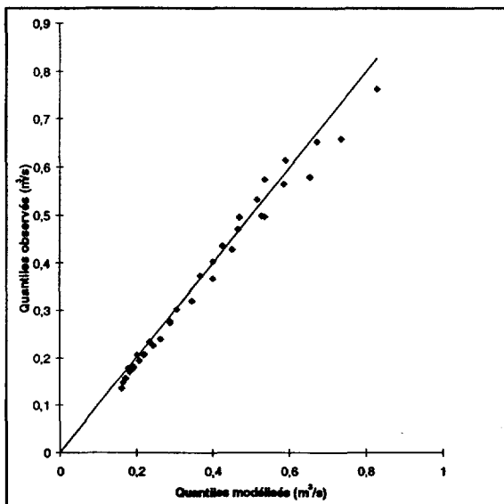
Figure 23 Banestilor à HALMAGIU « QCN(T, d) ». Banestilor's basin at HALMAGIU "QCN(T, d)". ( D_e = 8,8 j et VCN(2, 1) = 0,278 m 3 /s) – Nash% : 97,5.
