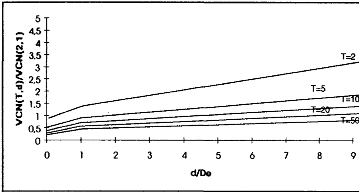
Figure 6 Abaqués années sèches Vaubarlet. Standardized curves of Vaubarlet for dry years
