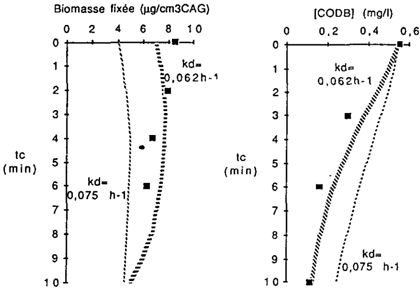
Figure 4 Superposition des concentrations en CODB(BL) et en biomasse fixée (■) mesurées dans le filtre 56 (hauteur du CAG = 2,5 m ; vitesse de filtration 15 m/h, donc temps de contact de 10 min ; T = 18,6 °C) et de la simulation calculée par le modèle CHABROL pour deux valeurs du taux de mortalité ( k_d ). Profil relevé six mois après la mise en service du filtre.
