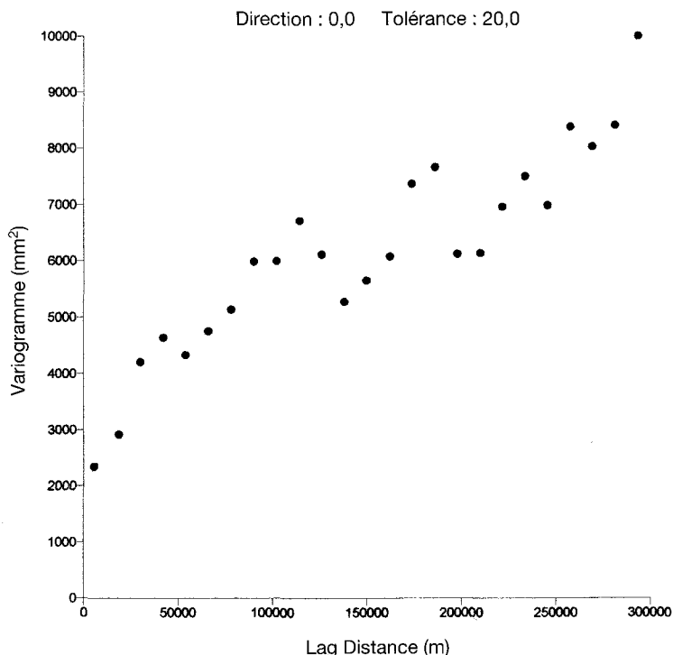
Figure 15 Variogramme multidirectionnel des précipitations interannuelles moyennes ramenées à une altitude de 1 000 m, pour la RH36 seulement.
