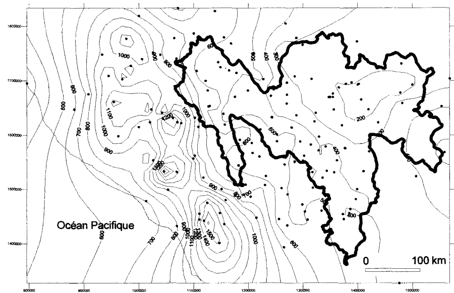
Figure 4 Isohyètes interannuelles et localisation des postes pluviométriques dans le bassin Nazas-Aguanaval et ses environs. Interannual isohyets and location of rain gauges in the Nazas-Aguanaval basin and surrounding areas.
