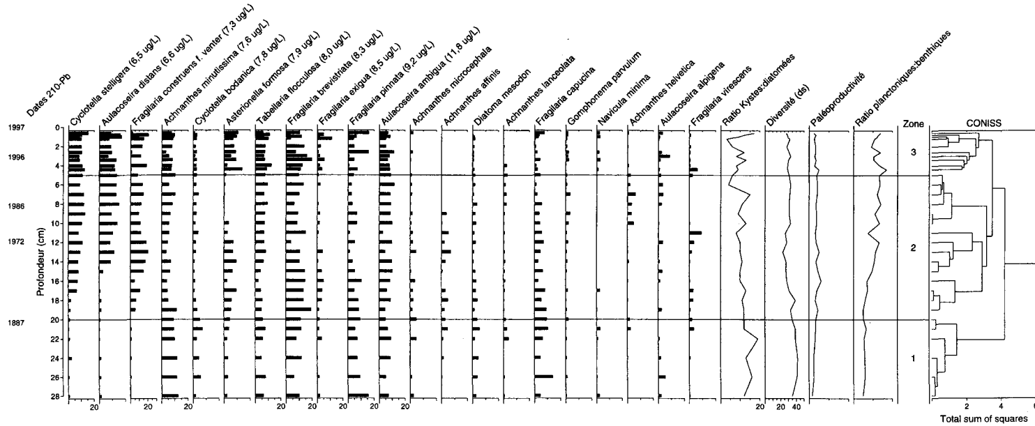
Figure 6 Diatomées dominantes, ratio espèces planctoniques : benthiques ( 10^{-1} ), paléoproduktivité ( \times 10^7 ), ratio kystes : diatomées ( 10^{-2} ) et la diversité ( d_s ) dans les sédiments du lac Saint-Charles. L'optimum de P ( \mu\text{g}\cdot\text{L}^{-1} ; HALL et SMOL, 1996) est indiqué pour chaque espèce de diatomée.
