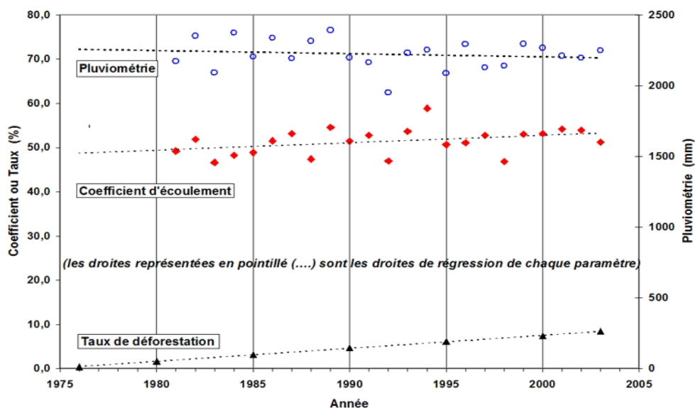
Figure 6. Période 1981-2003. Évolution dans le temps de la pluviométrie moyenne annuelle, du coefficient d'écoulement et du taux de déboisement.
