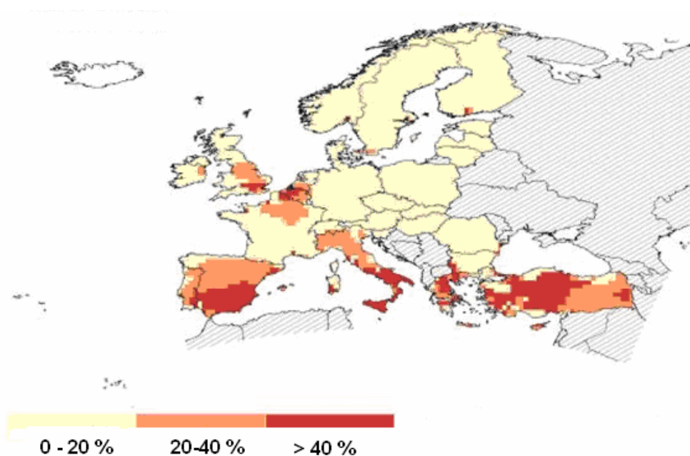
Figure 8. Taux de pénurie en eau en Europe en 2030, d'après ECOLOGIC (2007) et Center for Environmental Systems Research, University of Kassel, August 2004, WaterGAP 2.1e. Rapport prélèvements sur disponibilité par bassin, scénario de base LREM-E. Water stress ratio in Europe in 2030, from ECOLOGIC (2007) and Center for Environmental Systems Research, University of Kassel, August 2004, WaterGAP 2.1e. Withdrawal-to-availability ratio per basin, baseline LREM-E scenario.
