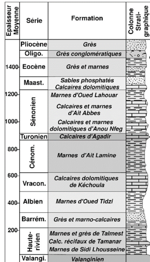
Figure 2. Coupe stratigraphique synthétique du Crétacé et du Tertiaire de la zone d'étude. Le symbole —●— représente les systèmes aquifères de la partie aval et —★— les systèmes aquifères de la partie amont du bassin d'Essaouira.
