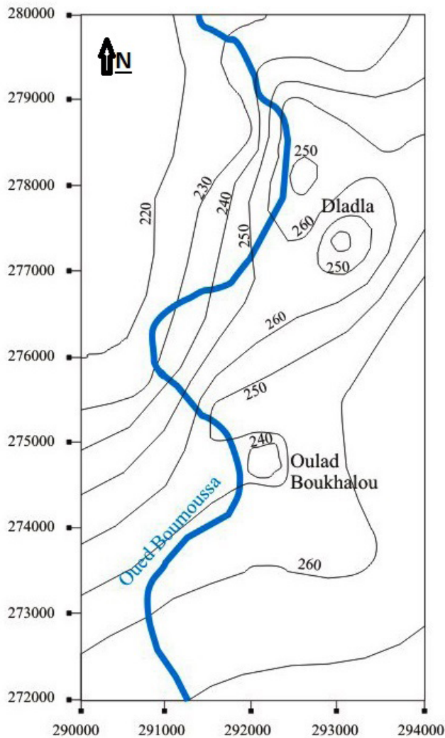
Figure 2. Carte piézométrique de janvier 2004 (EL AMRANI et al., 2008). Carte en coordonnées Lambert; les lignes noires sont des courbes isopièzes (m asl). Piezometric map of January 2004 (EL AMRANI et al., 2008). Map in Lambert coordinates; black lines correspond to piezometric levels (m asl).
