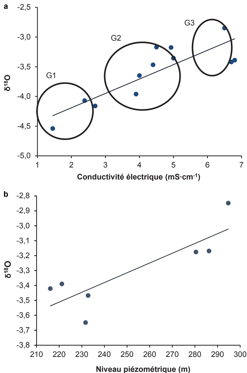
Figure 7. Relations entre les compositions en \delta^{18}\text{O} et a) les conductivités électriques et b) les niveaux piézométriques. G1 : échantillons pris dans les puits profonds (Cénomanien) qui sont moins enrichis en \delta^{18}\text{O} ; G2 : échantillons pris dans les puits superficiels (Plioquaternaire) plus enrichis en \delta^{18}\text{O} (évaporation et mélange) et G3 : échantillons du Plioquaternaire, plus enrichis en \delta^{18}\text{O} et aux valeurs de conductivité électrique les plus élevées. Relationship between compositions in \delta^{18}\text{O} and a) electrical conductivity and b) piezometric levels. G1: samples taken in deep wells (Cenomanian) which are less enriched in \delta^{18}\text{O} ; G2: samples taken from superficial wells (Plioquaternary) enriched in \delta^{18}\text{O} (evaporation and mixing) and G3: Plioquaternary samples, more enriched in \delta^{18}\text{O} and with the highest electrical conductivity.
