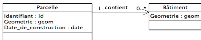
Figure 4. Diagramme simplifié des données cadastrales utilisées.
