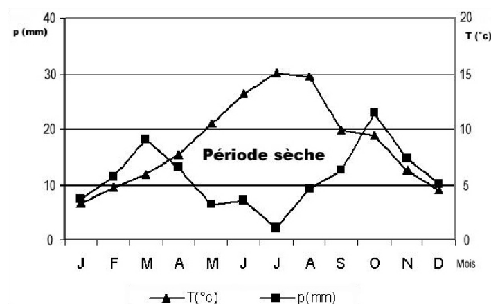
Figure 8. Diagramme Ombrothermique (1990-2002).
