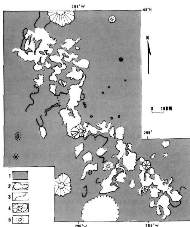
FIGURE 7. Dépressions coalescentes sur Mars au nord de Isidis Planitia: 1) plaine sédimentaire récente; 2) alas; 3) talus; 4) cratère d'impact à éjectas lobés; 5) buttes résiduelles.
