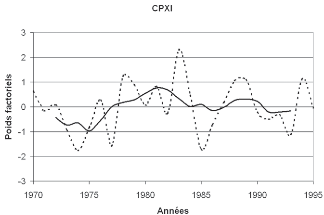
FIGURE 5. Variabilité interannuelle des poids factoriels des composantes principales qui forment le mode III. La courbe en gras représente les valeurs lissées des notes factorielles.
