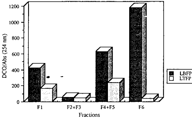
Figure 3 Comparaison des rapports DCO/Abs des différentes fractions des lixiviats de FOUSSAIS-PAYRE.
