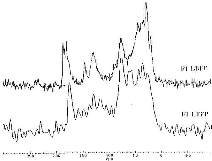
Figure 5 Spectres RMN C^{13} des fractions F1 du lixiviat brut de FOUSSAIS-PAYRE (F1 LBFP) et traité (F1 LTFP).
