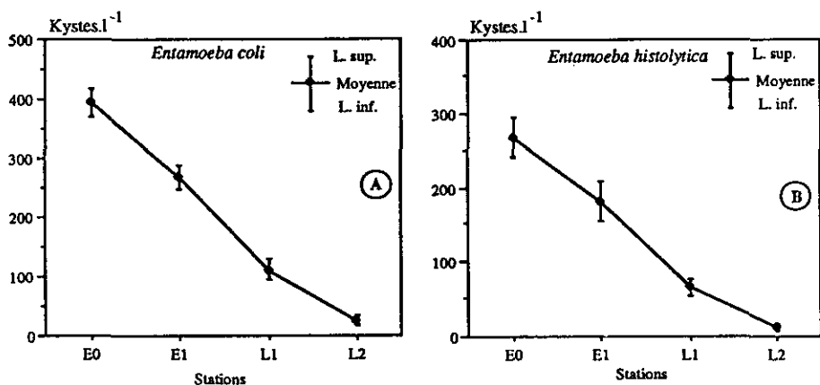
Figure 5 Évolution temporelle des concentrations des kystes d' E. coli (A) et d' E. histolytica (B) dans les eaux usées brutes (E0) et dans les eaux épurées (L2) par lagunage.
