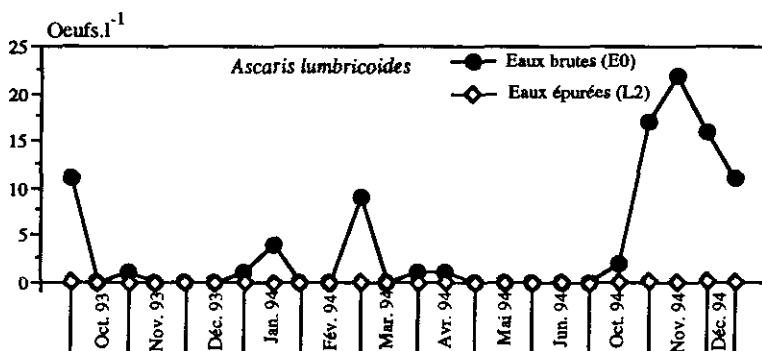
Figure 7 Évolution temporelle des concentrations des œufs d' Ascaris lumbricoides dans les eaux usées brutes (E0) et dans les eaux usées épurées (L2) par lagunage.
