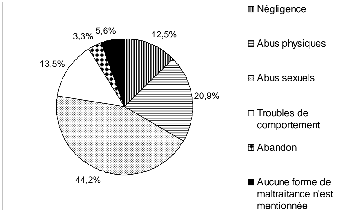
Figure 2 : Répartition de l'ensemble des problématiques mentionnées dans les articles en 2004-2006 (N = 665)
