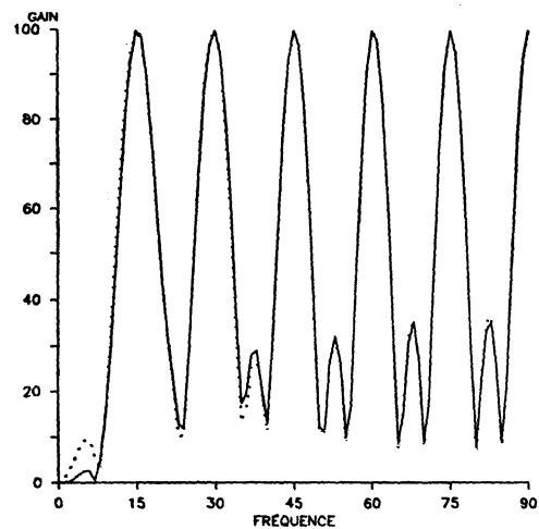
Figure 13 Gains saisonniers relatifs à la 35-ième période d'estimation du X-11-ARMMI triennial standard (.....) et à poids cyclo-tendanciels optionnels (—)
