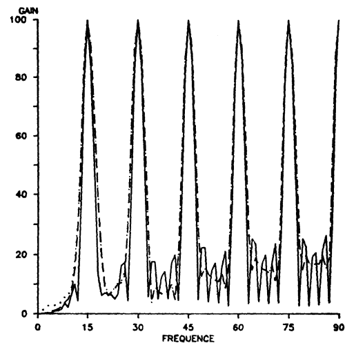
Figure 2. Gains saisonniers relatifs à la 71-ième période d'estimation du X-11-ARMMI septennal standard (.....), à poids cyclo-tendanciels optionnels (---) et à poids cyclo-tendanciels optionnels et saisonniers proposés (—)
