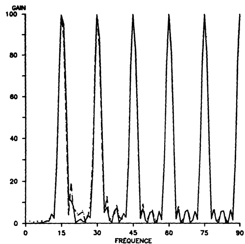
Figure 1. Gains saisonniers relatifs à la 43-ième période d'estimation du X-11-ARMMI septennal standard (.....), à poids cyclo-tendanciels optionnels (---) et à poids cyclo-tendanciels optionnels et saisonniers proposés (—)
