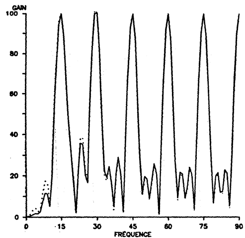
Figure 9 Gains saisonniers relatifs à la 25-ième période d'estimation du X-11-ARMMI quadriennal standard (.....) et à poids cyclo-tendanciels optionnels (—)
