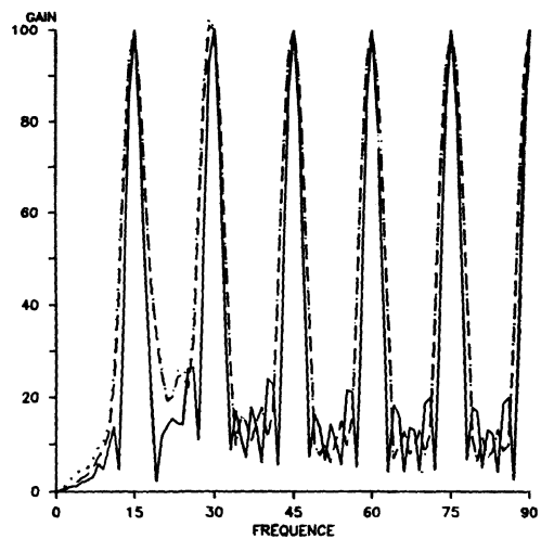
Figure 5. Gains saisonniers relatifs à la 84-ième période d'estimation du X-11-ARMMI septennal standard (.....), à poids cyclo-tendanciel optionnels (---) et à poids cyclo-tendanciel optionnels et saisonniers proposés (—)
