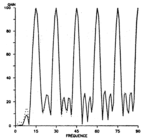
Figure 10 Gains saisonniers relatifs à la 47-ième période d'estimation du X-11-ARMMI quadriennal standard (.....) et à poids cyclo-tendanciels optionnels (—)
