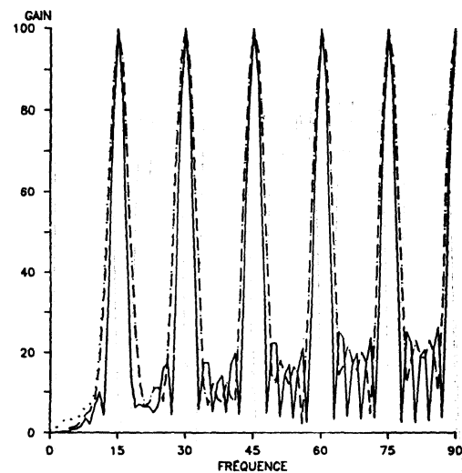
Figure 4 Gains saisonniers relatifs à la 83-ième période d'estimation du X-11-ARMMI septennal standard (·····), à poids cyclo-tendanciels optionnels (---) et à poids cyclo-tendanciels optionnels et saisonniers proposés (—)
