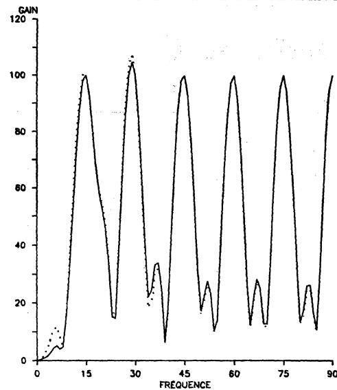
Figure 14 Gains saisonniers relatifs à la 36-ième période d'estimation du X-11-ARMMI triennial standard (.....) et à poids cyclo-tendanciels optionnels (—)
