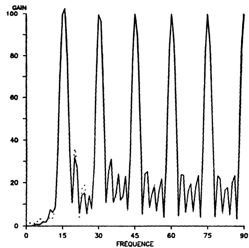
Figure 6. Gains saisonniers relatifs à la 31-ième période d'estimation du X-11-ARMMI quinquennal standard (.....), à poids cyclo-tendanciel optionnels (---) et à poids cyclo-tendanciel optionnels et saisonniers proposés (—)
