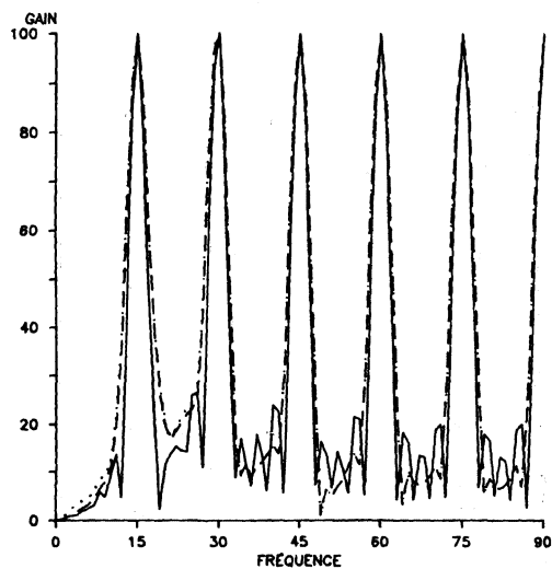
Figure 3 Gains saisonniers relatifs à la 72-ième période d'estimation du X-11-ARMMI septennal standard (·····), à poids cyclo-tendanciels optionnels (---) et à poids cyclo-tendanciels optionnels et saisonniers proposés (—)
