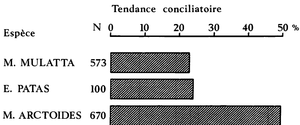
Figure 3 : Tendance conciliatoire définie comme le pourcentage d'adversaires mutuellement attirés (voir texte). Les données portent sur trois espèces de singes captifs et proviennent d'observations d'une durée de dix minutes par de Waal et Yoshihara (1983), York et Rowell (1988), et de Waal et Ren (1988). N est l'échantillon total de paires d'adversaires.
