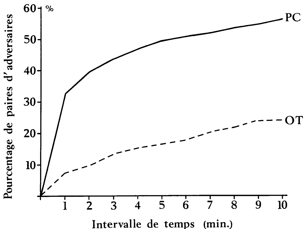
Figure 2 : Pourcentage cumulatif de paires d'adversaires établissant des contacts corporels post-conflituels (PC) ou pendant les observations témoins (OT) dans un groupe de macaques à queue tronquée (de Waal et Ren 1988).
