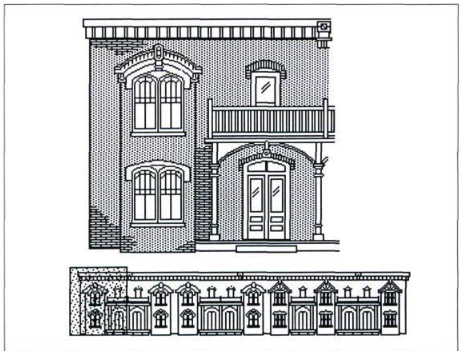
Schéma d'une maison vernaculaire en rangée ou en bande: 566-607, rue Prospect, Sherbrooke. Infographie: Gaéтан Bousquet, 1988.
