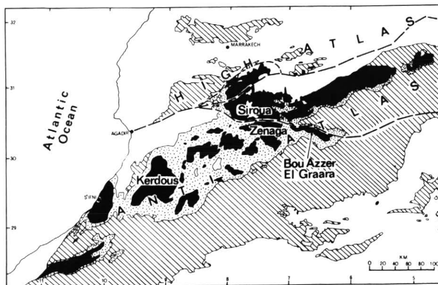
Figure 1 Localisation des boutonnières Précambriennes de l'Anti-Atlas du Maroc. Blanc—couverture Secondaire et Tertiaire; hachures—Primaire (sauf le Cambrien Intérieur du domaine de l'Anti-Atlas); pointillé—Cambrien Intérieur et Adoudounien du domaine de l'Anti-Atlas; noir—Précambrien.
