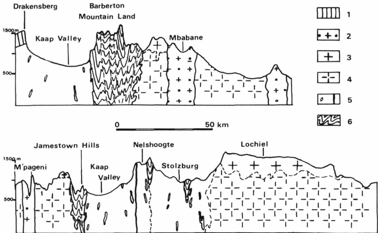
FIGURE 9. D'après M.J. et R.P. VILJOEN (1970). 1) Quartzite du Black Reef. 2) Granite des «jeunes plutons». 3) Granite de coupole. 4) Gneiss et migmatites infragranitiques. 5) Granodiorites (avec xénolites d'Onverwag et dykes basiques). 6) Formations paramétamorphiques du système du Swaziland.
