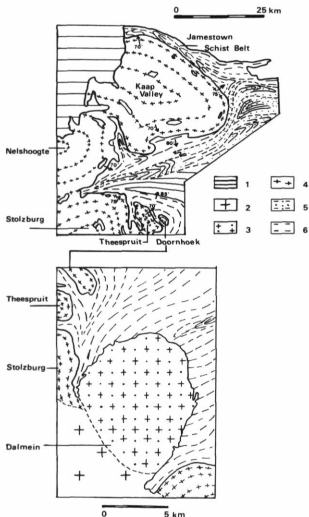
FIGURES 6 et 7. D'après M. J. et R. P. VILJOEN (1970). 1) Système du Transvaal. 2) Granite de coupole. 3) Granite des «vieux plutons». 4) Granodiorite (à biotite ou à hornblende). 5) Groupes de Fig Tree et de Moodies. 6) Groupe d'Onverweg
