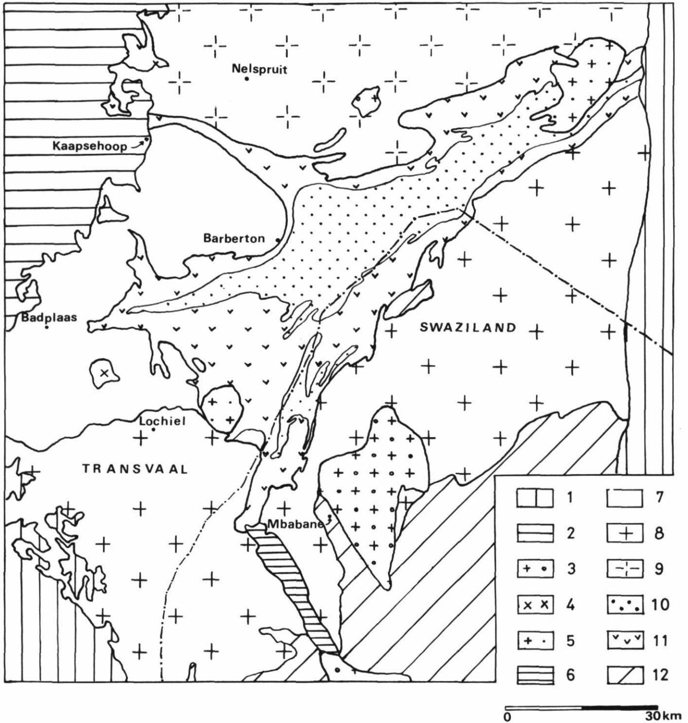
FIGURE 5. D'après M. J. et R. P. VILJOEN (1970) et HUNTER (1973). 1. Sédiments du système Karoo. 2) Sédiments du système du Transvaal. 3) Granite des «jeunes plutons». 4) Syénite de Bosmankop. 5) Granite des «vieux plutons». 6) Formations paramétamorphiques du système de Pongola. 7) Granodiorite. 8) Granite de coupole. 9) Gneiss et migmatites de Nelspruit. 10) Formations para-métamorphiques des groupes de Fig Tree et de Moodies. 11) Formations paramétamorphiques du groupe d'Onverwag. 12) Gneiss du Basement Complex.
