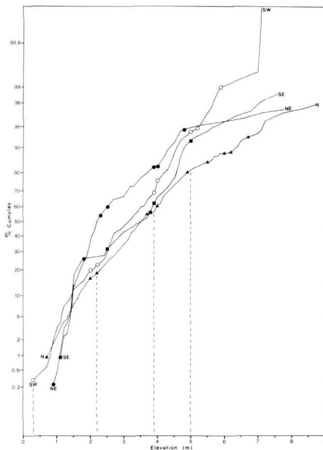
FIGURE 9. Regroupement des niveaux d'aplanissement selon les courbes des fréquences cumulées des altitudes sur les profils des plates-formes.
