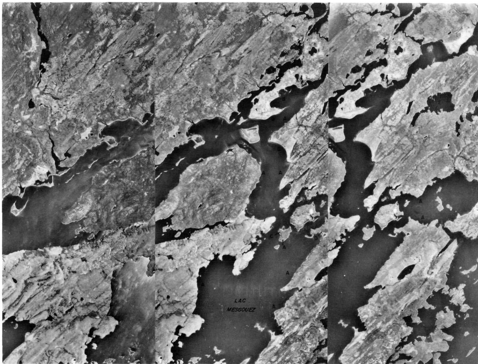
FIGURE 12. Paysage de la région des nombreux lacs de l'est. Les importantes fluctuations du niveau de l'eau (de l'ordre de 2 m) du lac Mesgouez permettent la formation d'une rive étroite sur matériel grossier (A). Dans la partie supérieure du lac, les dépôts fluvio-glaciaires favorisent le développement d'une rive étroite sur matériel moyen (B). Face aux vents dominants, on note la présence de plages (C) et de tourbières érodées (D). Enfin, la rive très étroite (E) ceinture un petit lac situé à la droite du lac Mesgouez (Photothèque nationale, Ottawa, A-15342, 22, 23 et 24; 19 juin 1956, 1/60 000).
