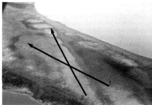
FIGURE 4. Superposition de deux directions d'écoulement glaciaire dans le till drumlinisé: 1) la plus ancienne, 2) la plus récente.
