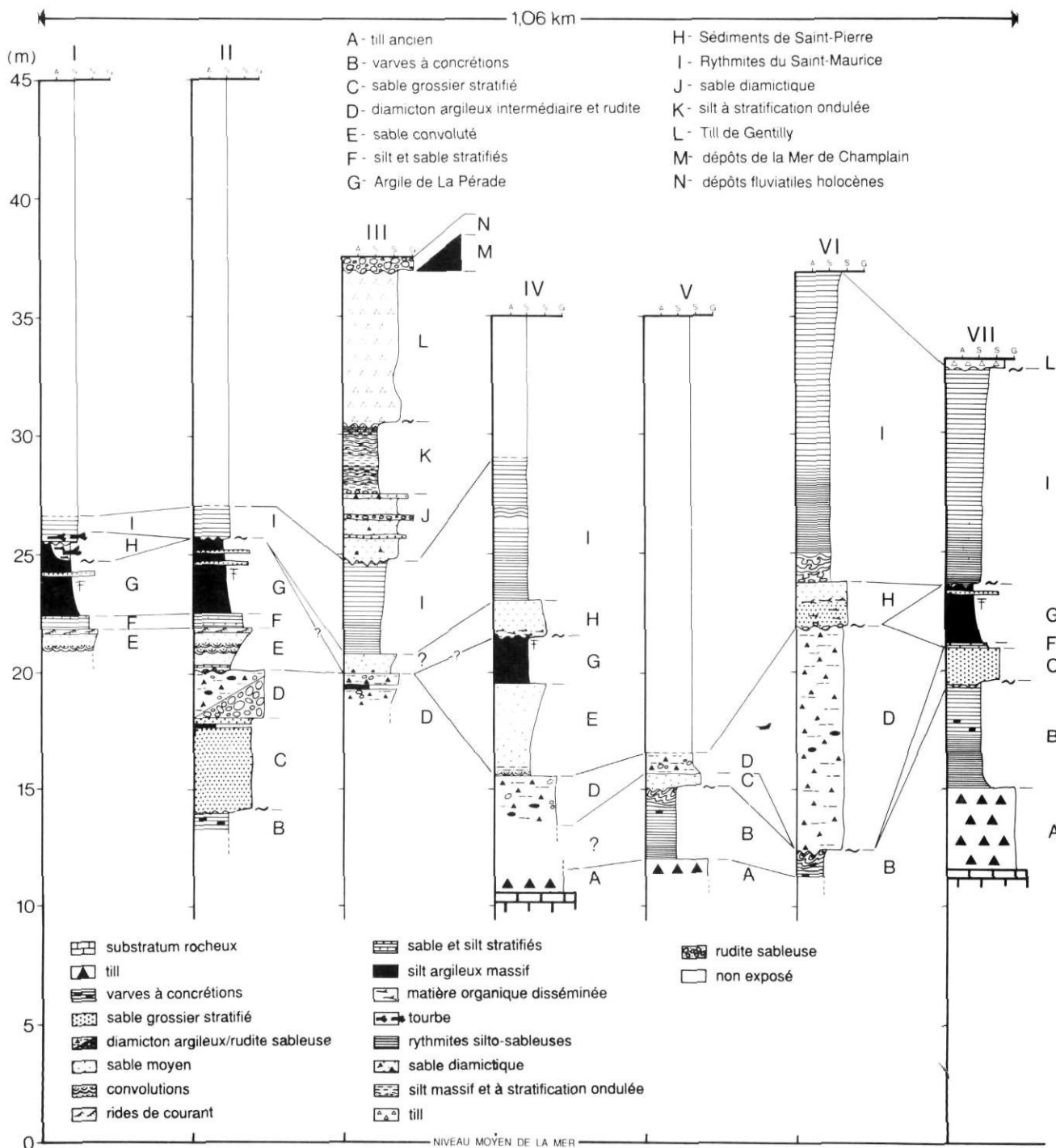
FIGURE 3. Corrélation entre les coupes I, II, III, IV, V, VI et VII de Sainte-Anne-de-la-Pérade (A = argile; S = silt; S = sable; G = gravier).
