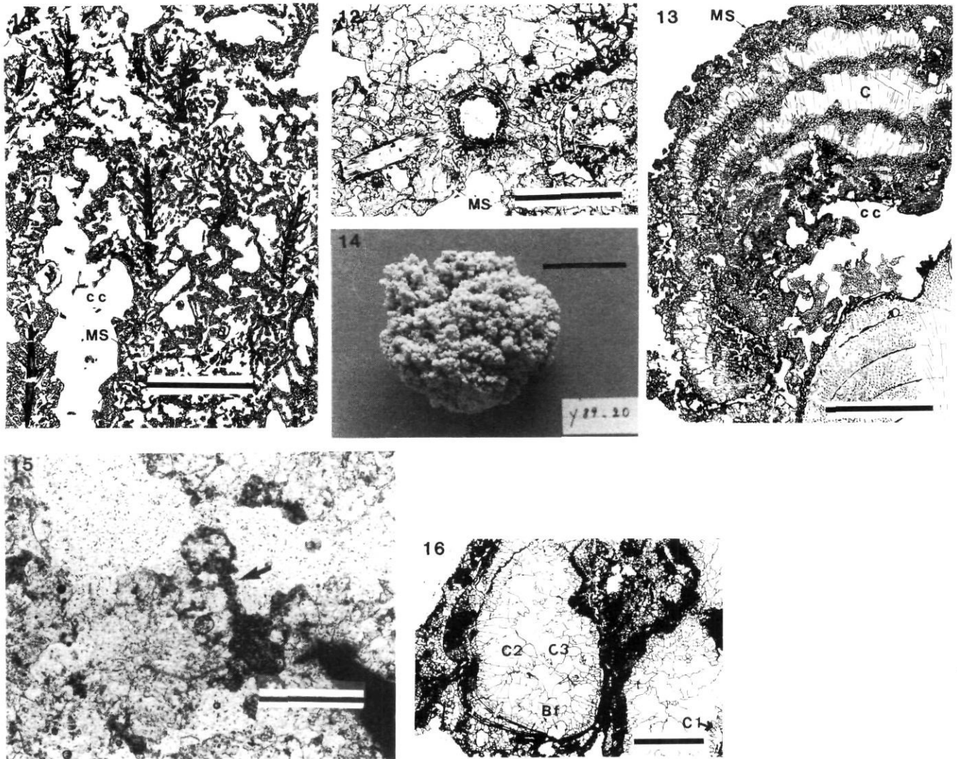
FIGURE 11. Dessin de l'échantillon Y.89-27 d'un sommet de barrage montrant des tiges et des feuilles de Bryum sp. recouvertes d'une trame microsparitique (MS). Minces ciments isopaches dans les cavités constitutionnelles (cc) indiquant un milieu phréatique (échelle: 4,3 mm).
