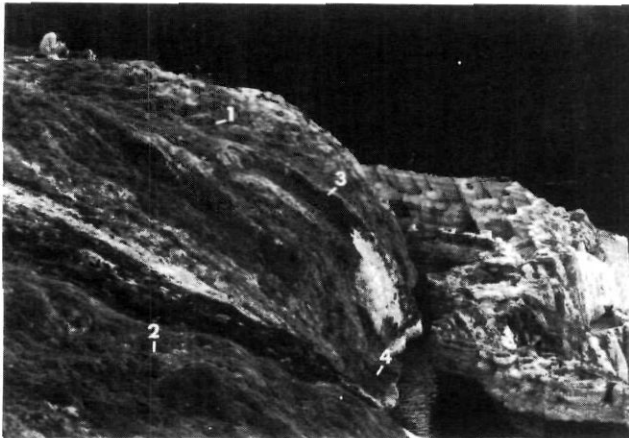
FIGURE 8. Étapes de l'épaississement d'une face aval de barrage: (1) cascates avec mini-barrages et mini-bassins; (2) mini-bassins couverts par les encroûtements successifs des mini-barrages; (3) évolution vers une convexité généralisée; (4) bassin entièrement recouvert par la progradation horizontale de la forme convexe, donnant une forme concave au pied du barrage.
