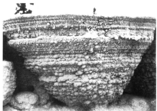
FIGURE 4. Un encorbellement de 60 cm de hauteur montrant des phases de croissance verticale et latérale, des phases de croissance verticale et des phases sans croissance. En haut, on voit un faciès tubulaire dans au moins trois couches; en bas, le faciès en glomérule cache le faciès tubulaire.
