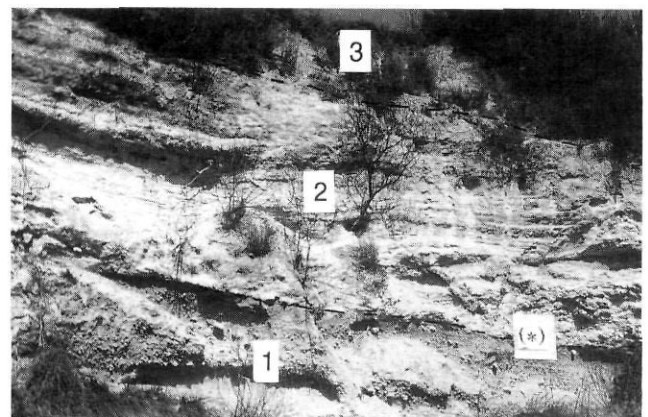
FIGURE 9. Coupe des travertins holocènes de Pont-de-Joux, rive droite de l'Huveaune. 1) niveaux détritiques, 2) tufs crayeux, 3) colluvions (* âge au ^{14}\text{C} de 7180 \pm 150 BP, Ly-4291).
