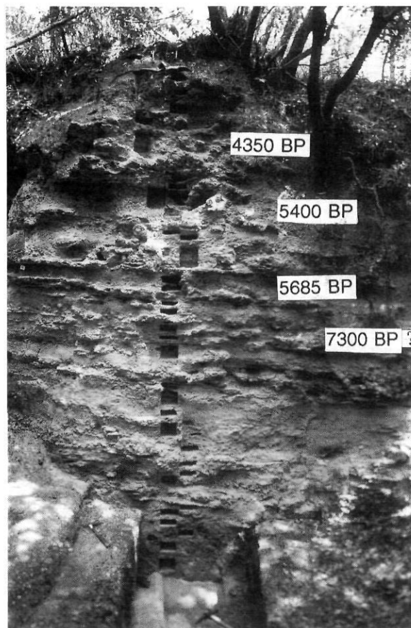
FIGURE 4. Les tufs du vallon de Jonquier (Salernes, Var). Coupe de Farizier (1980) et, dans la partie inférieure, sondage de Degaugue (1991). Alternance de faciès carbonatés clairs (« craies » et travertins) et de faciès colluviaux) ou anthropiques foncés.
