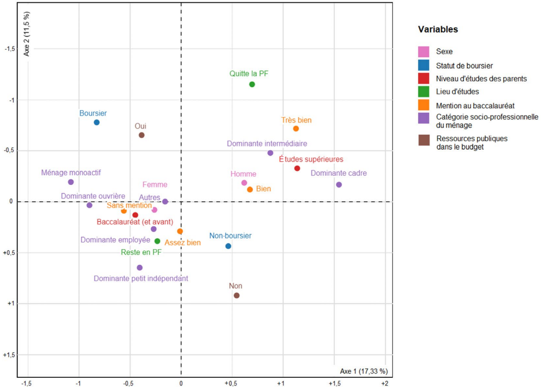
Graphique 2 Analyse des correspondances multiples (ACM)
