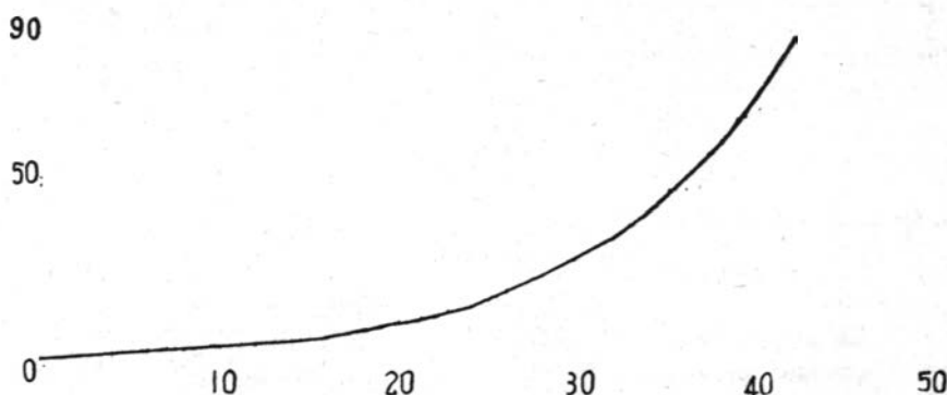
FIG. 7.—Courbe de l'équation: N = nht ; dans cette courbe et les suivantes, les ordonnées donnent le nombre des individus, les abscisses, le nombre de générations.
