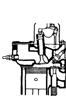
Moteur à soupapes en tête et arbre à cames dans le carter
