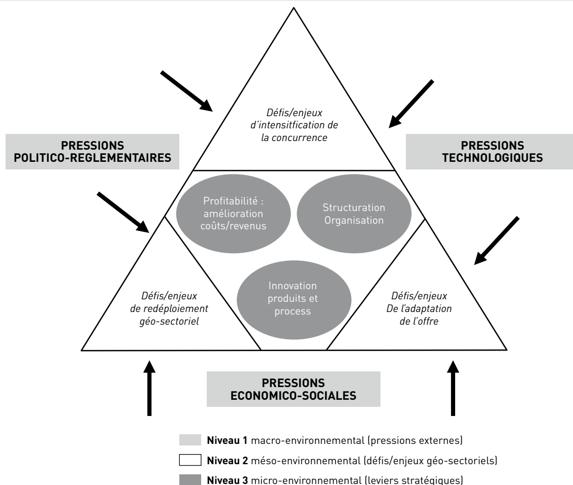
FIGURE 3 Le modèle PREST
