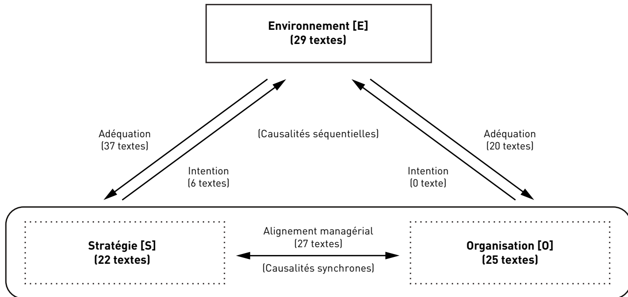
FIGURE 2 Le cadre ESO
