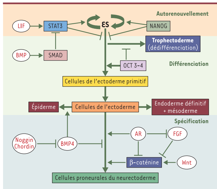
Figure 2. Pluripotentialité des cellules ES et induction de leur différenciation en cellules du neurectoderme. La prolifération des cellules ES est assurée par le facteur soluble LIF, au travers de l'activation de STAT3. De son côté, BMP active SMAD, qui inactive STAT3. NANOG intervient quant à lui en activant la prolifération des cellules ES et en inhibant leur différenciation. L'inactivation de STAT3, en l'absence de LIF, induit la différenciation des cellules ES en cellules de l'ectoderme primitif. En parallèle, OCT4, à une concentration basale, stimule l'autorenouvellement. Son absence entraîne en revanche la différenciation des cellules ES en trophoctoderme; à l'inverse, des doses élevées d'OCT4 induisent la différenciation des cellules ES en cellules de l'ectoderme primitif. L'inhibition de BMP4, grâce aux inhibiteurs naturels tels que Noggin et Chordin, induit la spécification neurale par défaut, au détriment de la différenciation épidermique. L'acide rétinoïque (AR) active la différenciation des cellules de l'ectoderme en neurectoderme au travers de deux mécanismes, l'un direct, l'autre via l'inhibition de la voie de signalisation Wnt/ \beta -caténine. Par ailleurs, l'acide rétinoïque inhibe aussi la voie de signalisation des FGF, connue pour sa régulation négative de la voie Wnt.
