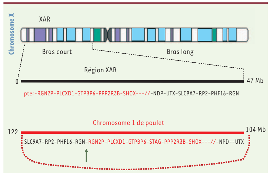
Figure 2. Homologie entre la région XAR de l'X humain et le chromosome 1 du poulet. Un chromosome en anneau hypothétique est représenté avec l'ordre des gènes observé chez le poulet par l'arc de cercle en rouge. Une recombinaison d'un tel anneau à l'extrémité du chromosome X en un point indiqué par la flèche verte pourrait expliquer la formation de la zone XAR en une seule étape (d'après [5]).
