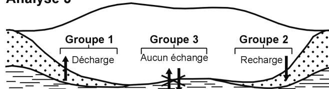
Figure 3. Représentation des groupes d'échange tourbière-aquifère utilisés pour identifier les espèces ou associations d'espèces indicatrices.
