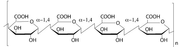
Figure 6. Structure d'un oligogalacturonate constitué d'une chaîne linéaire d'acides galacturoniques en \alpha -1,4. Les fragments les plus actifs ont, en général, un degré de polymérisation compris entre 11 et 14.
