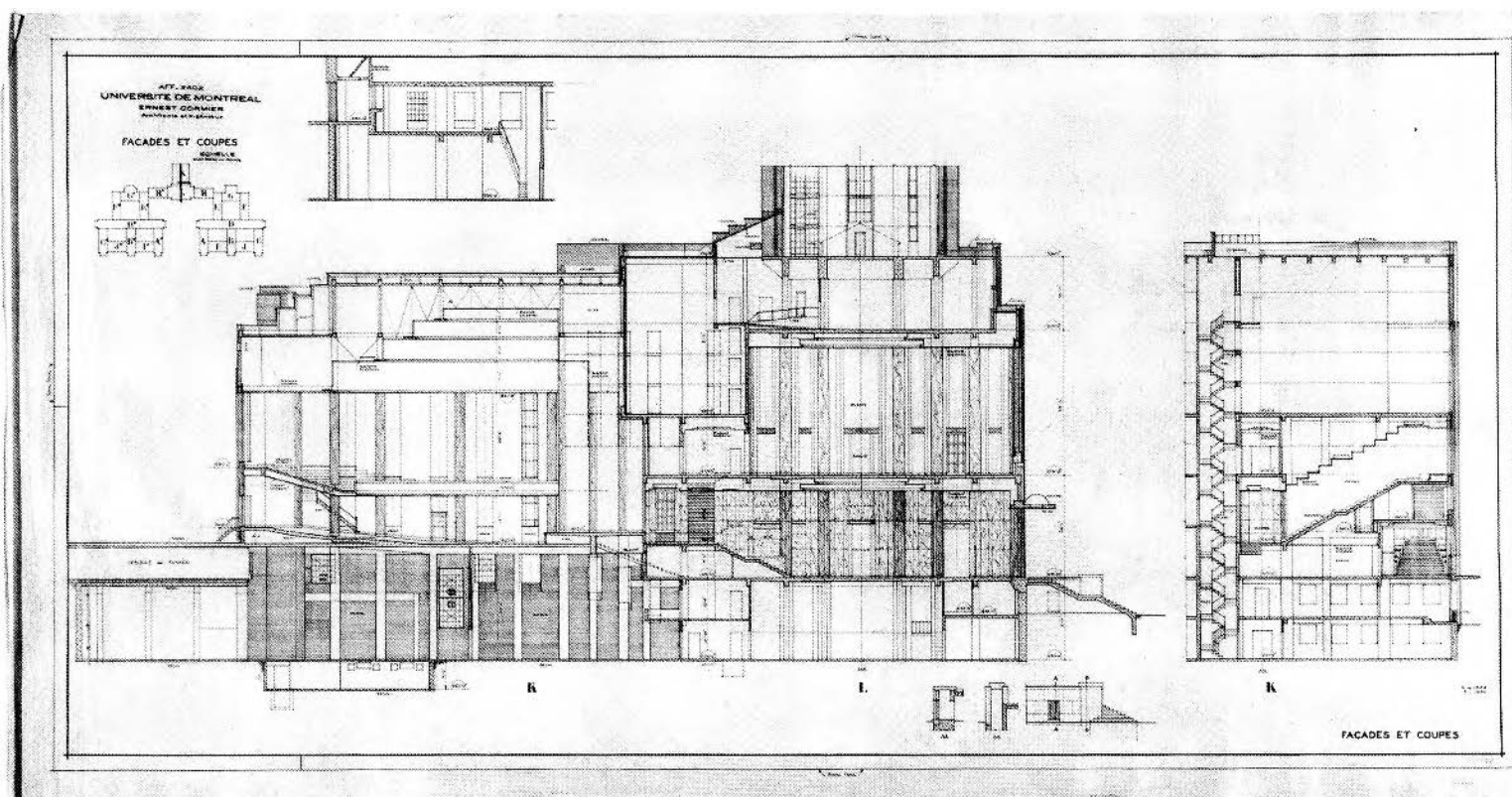
FIGURE 194. Ernest Cormier, Canada, Montréal 1885-Montréal 1980, Université de Montréal, coupe-façade sur le vestibule d'honneur et l'auditorium , encre sur toile, daté : 5 avril 1929 et 17 janvier 1930 », 65,6 × 138,3 cm. 01 Arc 141N, Collection Centre Canadien d'Architecture/Canadian Centre for Architecture, Montréal.
