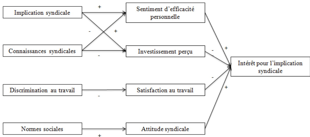
Figure 2. Modèle théorique
