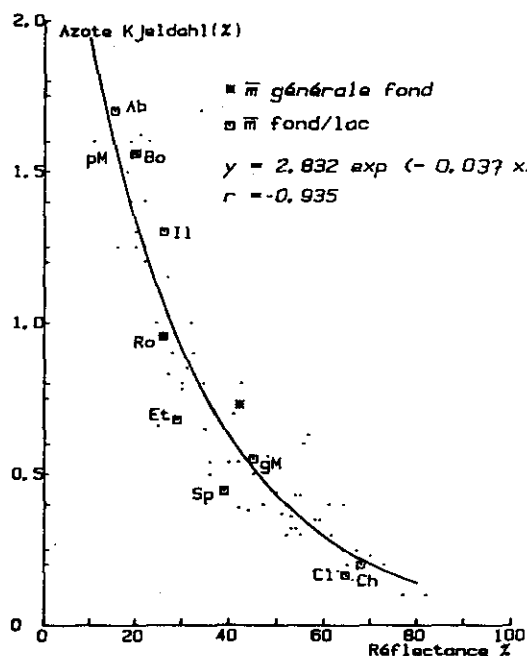
Figure 3.- Relation entre l'azote Kjeldahl et la "réflectance" pour dix lacs jurassiens.
