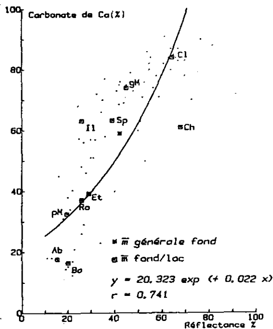
Figure 4.- Relation entre le carbonate de calcium et la "réflectance" pour dix lacs jurassiens.
