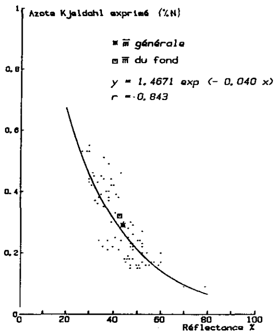
Figure 7.- Relation entre l'azote Kjeldahl et la "réflectance" pour le lac de Saint-Point.
