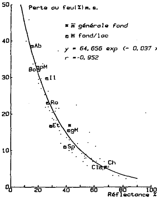
Figure 1.- Relation entre la perte au feu et la "réflectance" pour dix lacs jurassiens.
