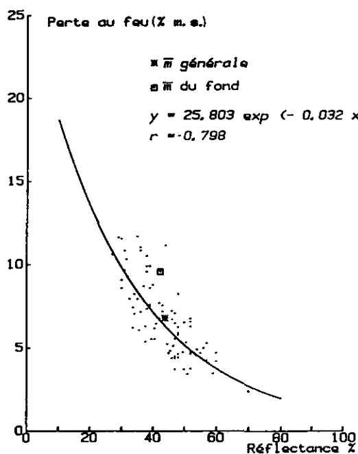
Figure 5.- Relation entre la perte au feu et la "réflectance" pour dix lacs jurassiens.
