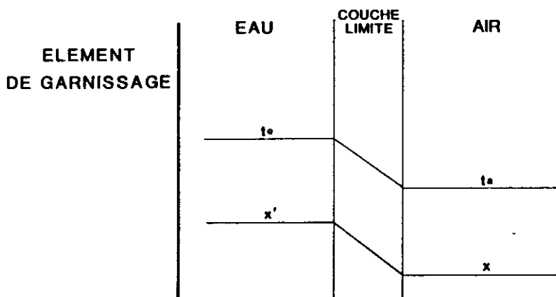
Figure 2 Schéma des échanges d'énergie et de matière à l'interface eau/air.
