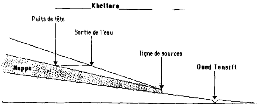
Principe de drainage de la nappe phréatique dans une Khattara
