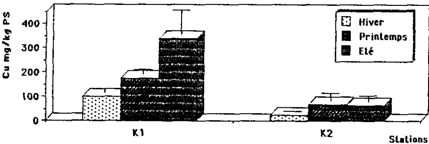
Figure 3 Évolution saisonnière du Cu chez M. praemorsa . Seasonal evolution of Cu in M. praemorsa .
