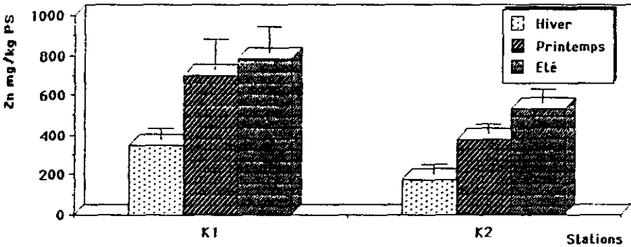
Figure 2 Évolution saisonnière du Zn chez M. praemorsa . Seasonal evolution of Zn in M. praemorsa .
