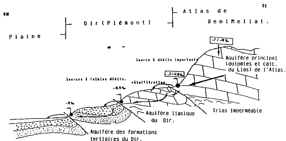
Figure 4 Schéma de circulation des eaux sur le piémont de l'Atlas de Beni Mellal. The water circulation diagram in piemont of Beni Mellal Atlas.
