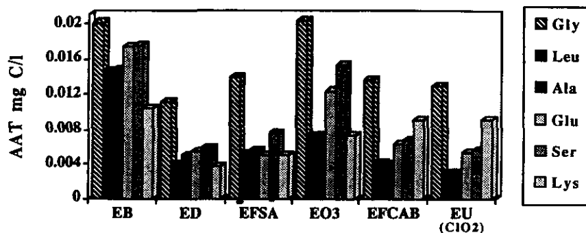
Figure 8a Evolution des acides aminés totaux prédominants dans la filière de traitement de l'usine de Ste-Rose durant la période d'été le 25.08.93 (EU : effluent usine post désinfecté au \text{ClO}_2 , autres abréviations : voir fig. 6).
