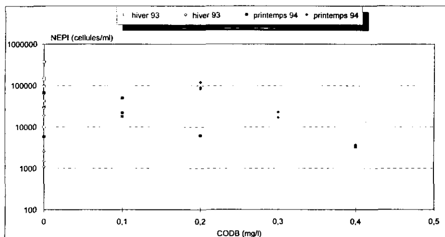
Figure 12 Evolution de la flore totale en fonction du CODB.
