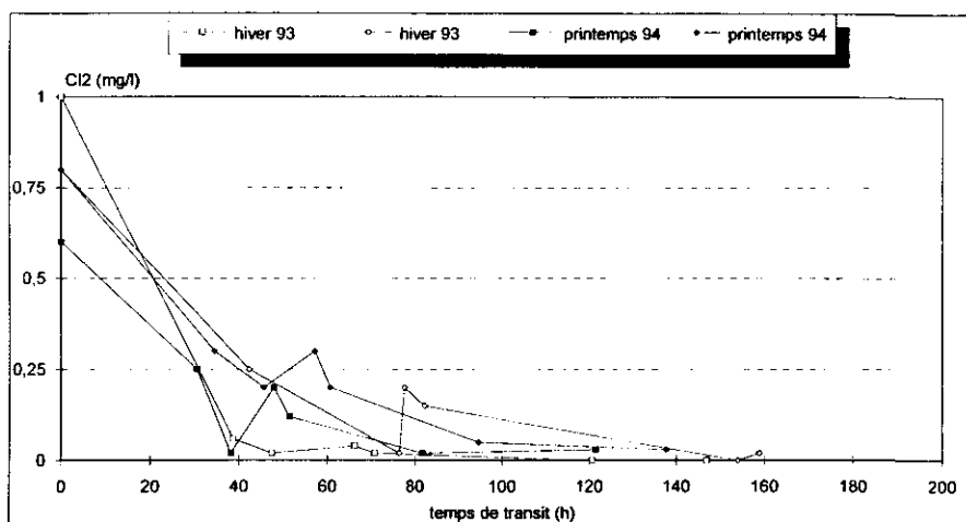
Figure 2 Evolution du désinfectant résiduel en fonction du temps de transit. Evolution of residual disinfectant as a function of residence time.
