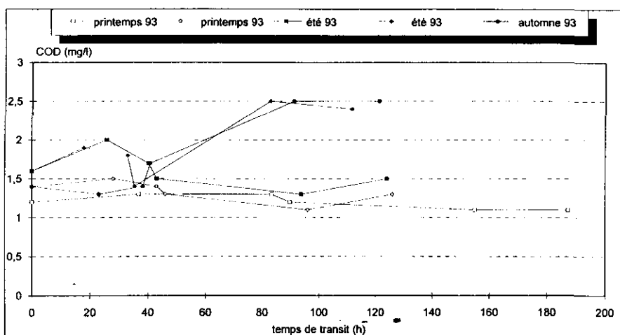
Figure 3 Evolution du COD en fonction du temps de transit : Série 1. Evolution of DOC as a function of residence time : Series 1.
