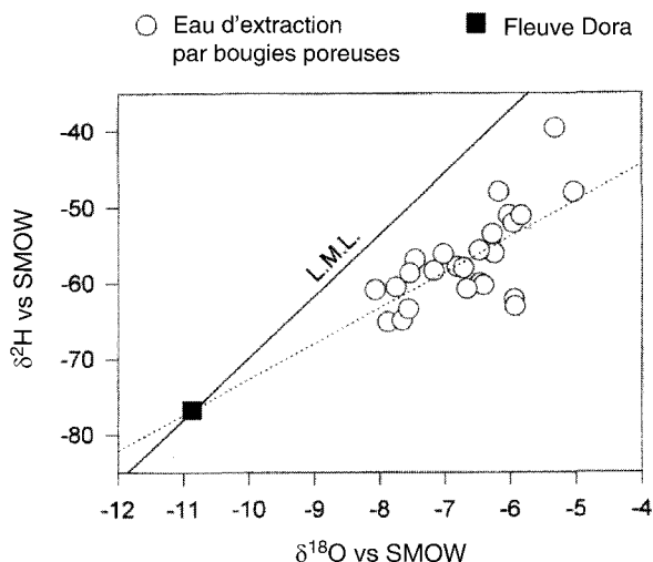
Figure 4 Composition isotopique des eaux d'extraction par bougies poreuses.
