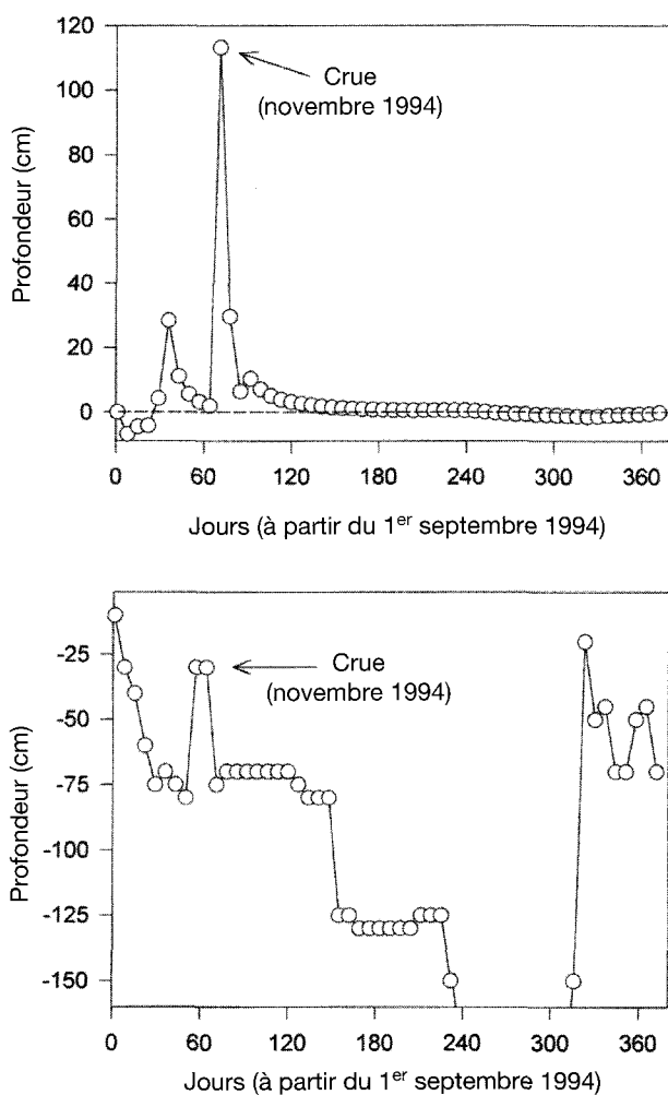
Figure 6 Recharge évaluée par la méthode du bilan hydrique et variation dans le temps de la profondeur du Plan de Flux Nul.
