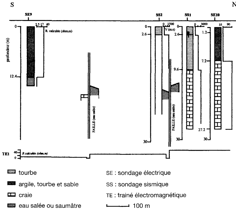
Figure 3 Essais géophysiques et leur traduction géologique le long du traîné électromagnétique TE1. Geophysical tests and their geological interpretation along electromagnetic profile TE1.
