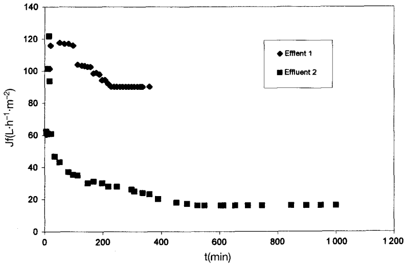
Figure 7a Variation du flux de filtration en fonction du temps pour les deux effluents à concentration variable ( P_{tm} = 2,2 \text{ bars} ; U = 3 \text{ m}\cdot\text{s}^{-1} et T = 43 \text{ }^\circ\text{C} ).
