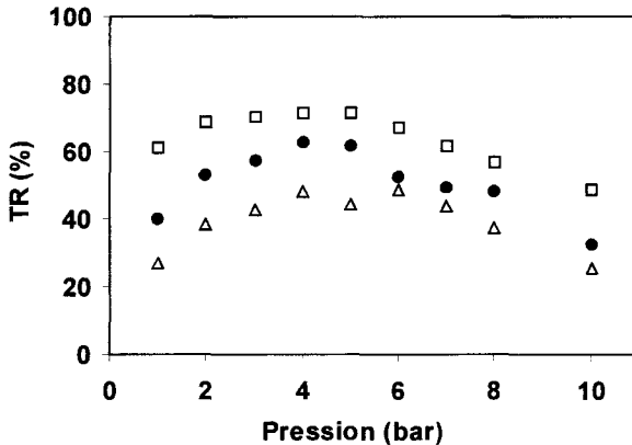
Figure 3 Variation du taux de rétention des nitrates en fonction de la pression pour trois concentrations différentes en \text{NH}_4\text{NO}_3 [□ 50, ● 100 et △ 200 \text{mg}(\text{NO}_3)\cdot\text{L}^{-1} ].
