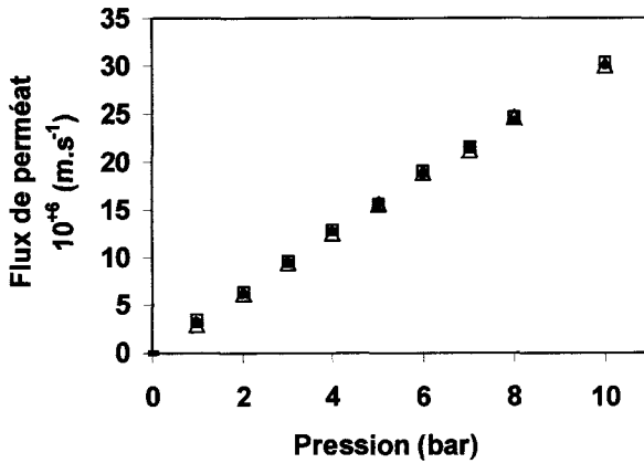
Figure 2 Variation du flux à l'eau (–) et du flux du perméat en fonction de la pression pour trois concentrations différentes en \text{NH}_4\text{NO}_3 [□ 50, ● 100 et △ 200 \text{mg}(\text{NO}_3)\cdot\text{L}^{-1} ].
