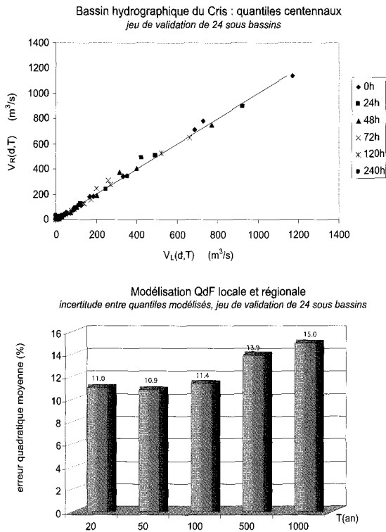
Figure 21 Validation du modèle régional, comparaison des quantiles 100 ans et graphe de synthèse. Regional model validation, 100-year quantiles comparison and synthesis graph.
