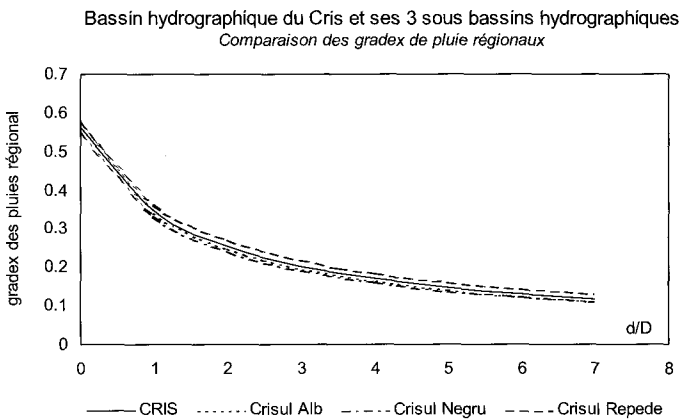
Figure 18 Comparaison des gradex de pluie régionaux. Regional rainfall gradex comparison.
