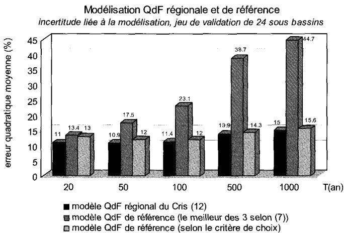
Figure 22 Comparaison des erreurs quadratiques moyennes des modèles QdF. Comparison of QdF models mean quadratic errors.
