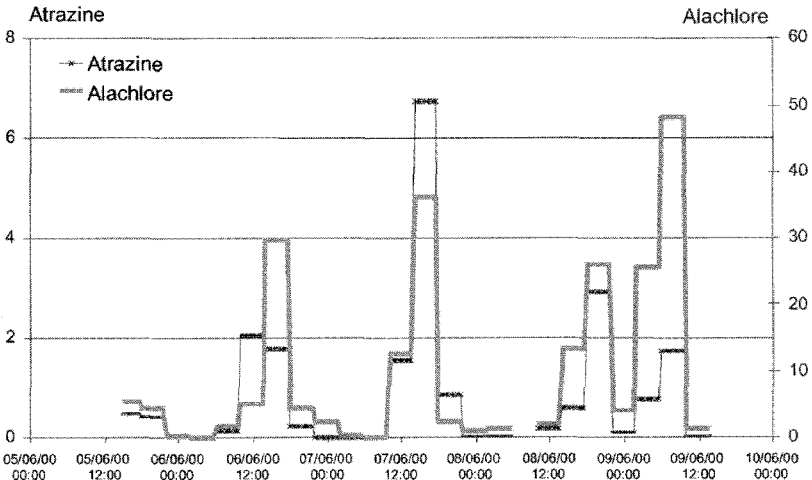
Figure 4 Flux de transferts vers l'atmosphère de l'atrazine et de l'alachlore appliqués sur une parcelle de maïs (juin 2000 ; BRIAND et al. , 2002).
